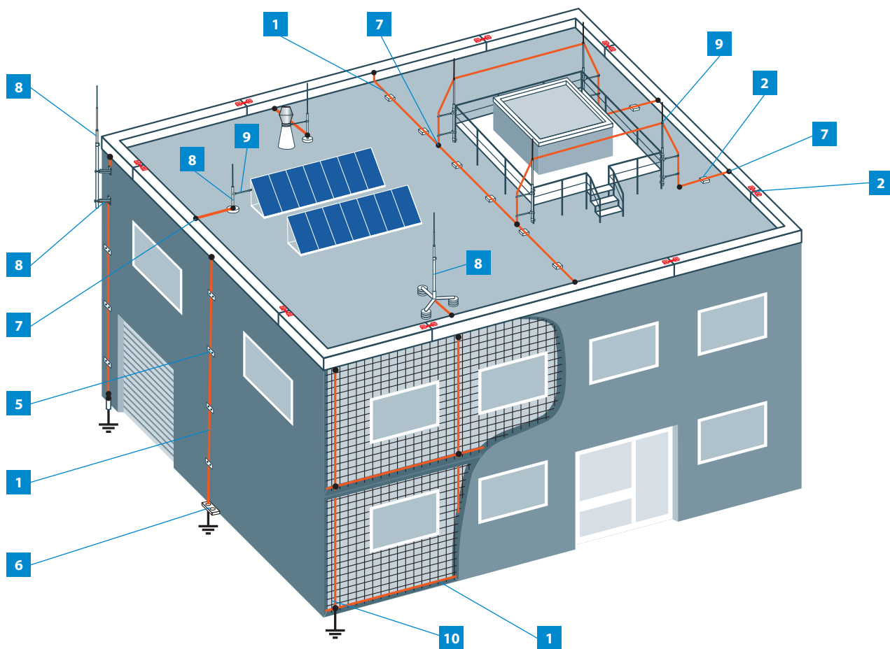
Внешняя система молниезащиты промышленного здания
