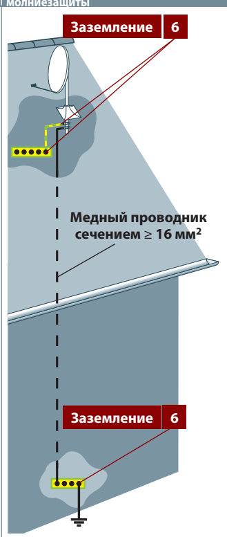
Уравнивание потенциалов внутри здания без внешней системы молниезащиты
