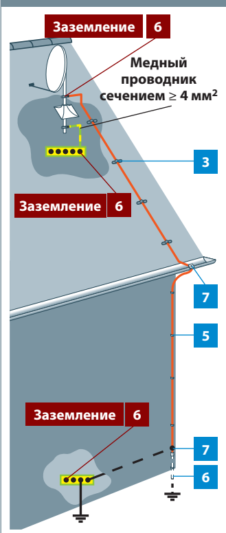
Уравнивание потенциалов вне здания без внешней системы молниезащиты
