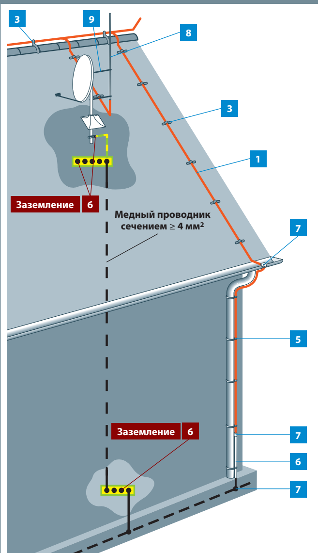
Уравнивание потенциалов вне здания без внешней системы молниезащиты
